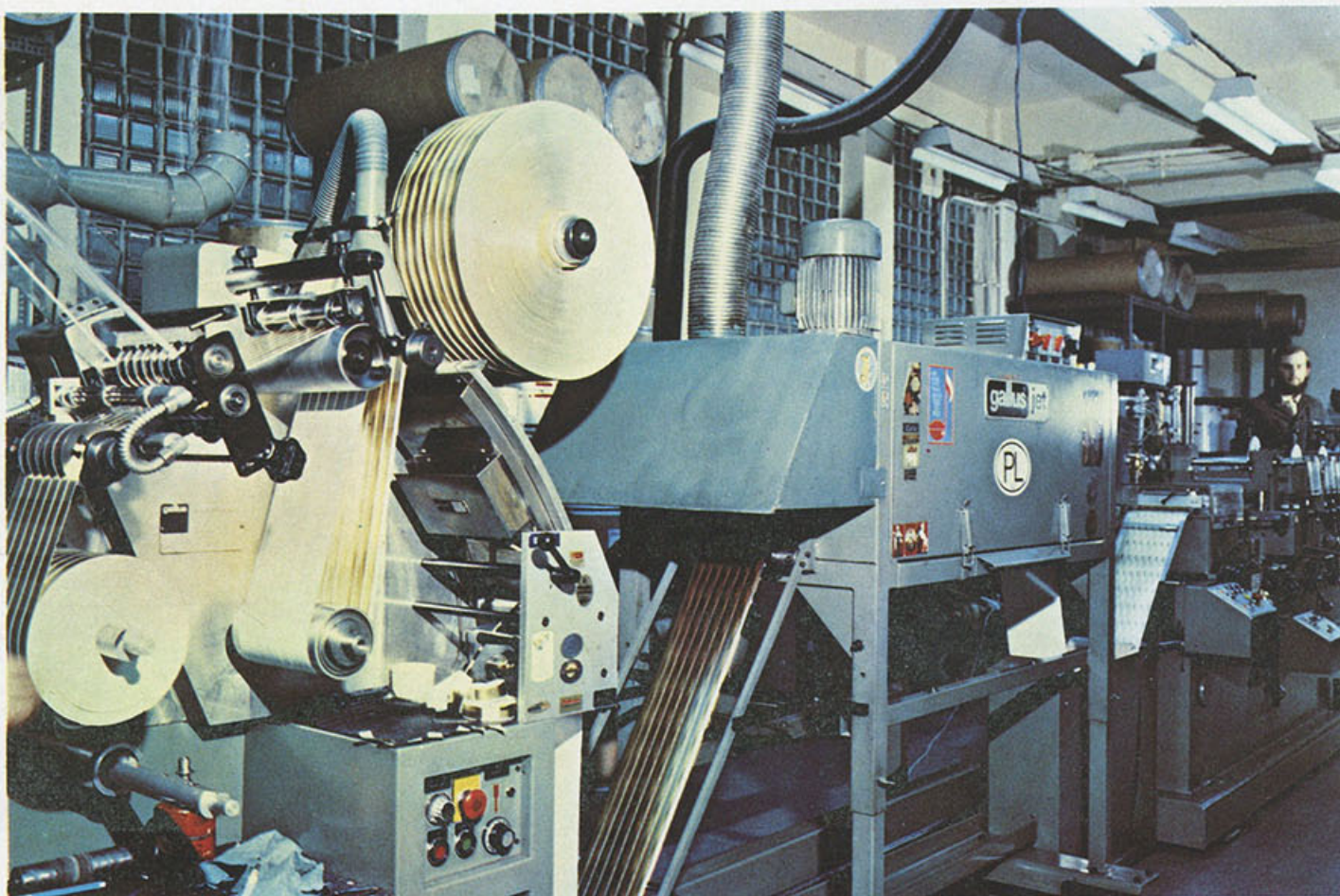
Maszyna do druku etykiet samoprzylepnych szwajcarskiej firmy Gallus
