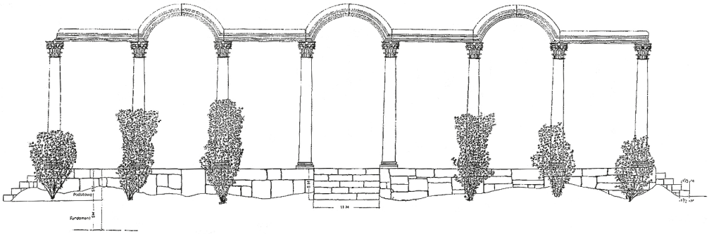
12. Rosarium w parku w Jabłonnej – Glorietta, projekt techniczny (konstrukcja); oprac. Mieczysław Kseniak, Lublin 2001 r.
